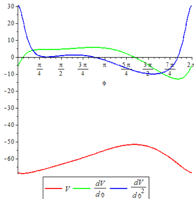
Rysunek 5: Energia potencjalna układu oraz jej pierwsza i druga pochodna w funkcji kąta \varphi , dla wybranej kombinacji ciężarków – Wxmaxima
