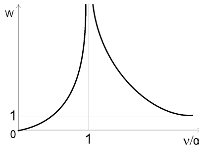
Rysunek 3: Wykres rezonansowy drgań wymuszanych bezwładnościowo
