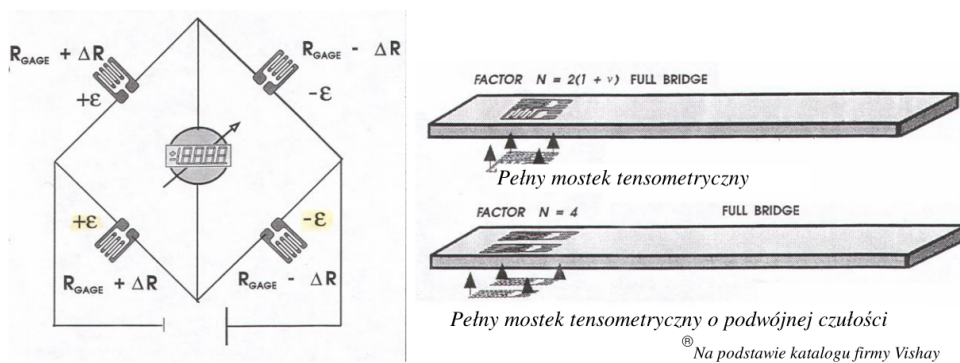
Rysunek 5: Tensometryczny mostek Wheatstone'a oraz sposób umieszczania tensometrów na pręcie
