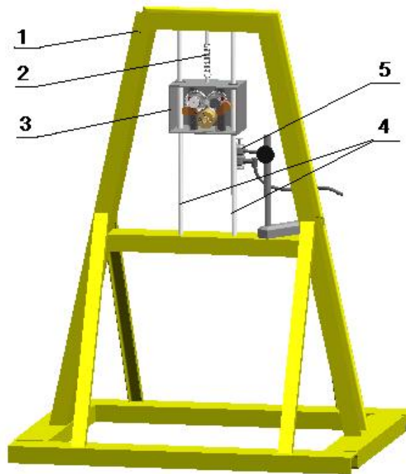
Rys.11.4. Stanowisko badawcze
