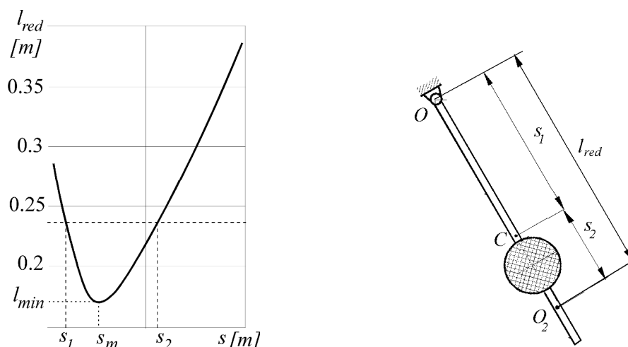
Rys. 5.2. Przebieg zmian długości zredukowanej wahadła ( l_{red} ) w funkcji odległości środka ciężkości wahadła od osi obrotu ( s )
