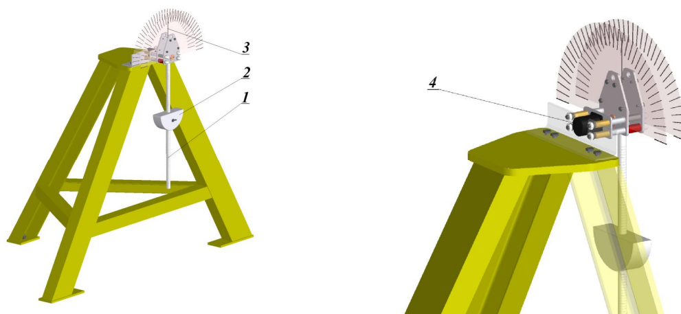
Rys. 5.5. Widok stanowiska pomiarowego
