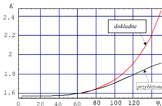
Rys. 5.4. Dokładna i przybliżona wartość całki eliptycznej ( K )
