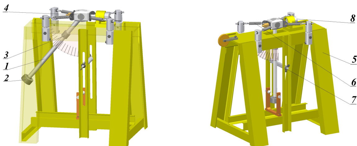
Rys. 6.2. Stanowisko badawcze
