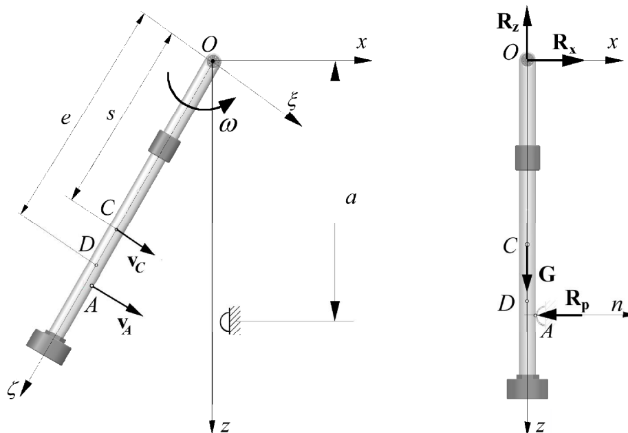
Rys. 6.1. Uderzenie mimośrodowe ciała nieswobodnego w nieruchomą przeszkodę:
